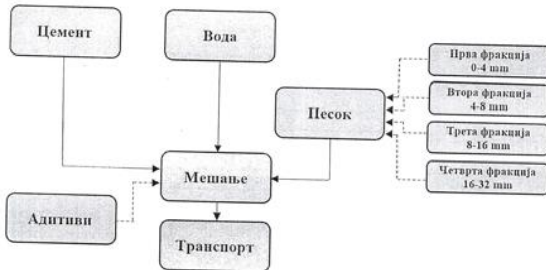
Слика бр.4 Процес на производство на бетон
