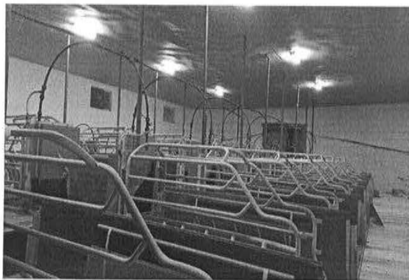
Сл.22 Систем за поење
